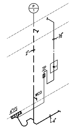
1 PLUMBING RISER DIAGRAM SCALE: NONE
