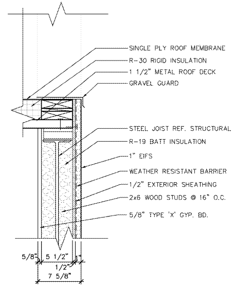
1 DETAIL SCALE: 1 1/2" = 1'-0"
