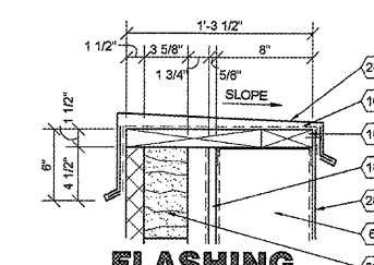
7 FLASHING SECTION A3.2 SCALE: 1 1/2" = 1'-0"
