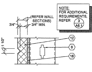
6 SECTION A3.2 SCALE: 1 1/2" = 1'-0"
