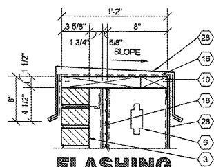
5 FLASHING SECTION A3.2 SCALE: 1 1/2" = 1'-0"
