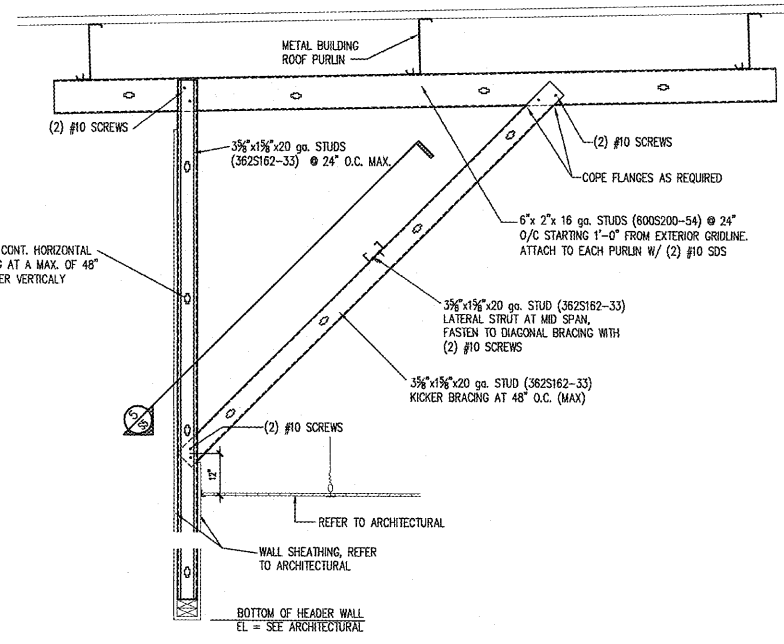
1 SECTION S5 SCALE: 3/4" = 1'-0"
