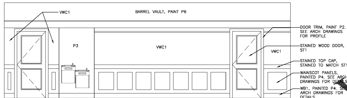
3 CORRIDOR C-1 ELEVATION - TYP. ID-3 SCALE: 3/8" = 1'-0"
