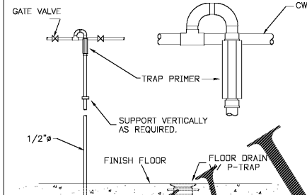
TRAP PRIMER DETAIL NO SCALE
