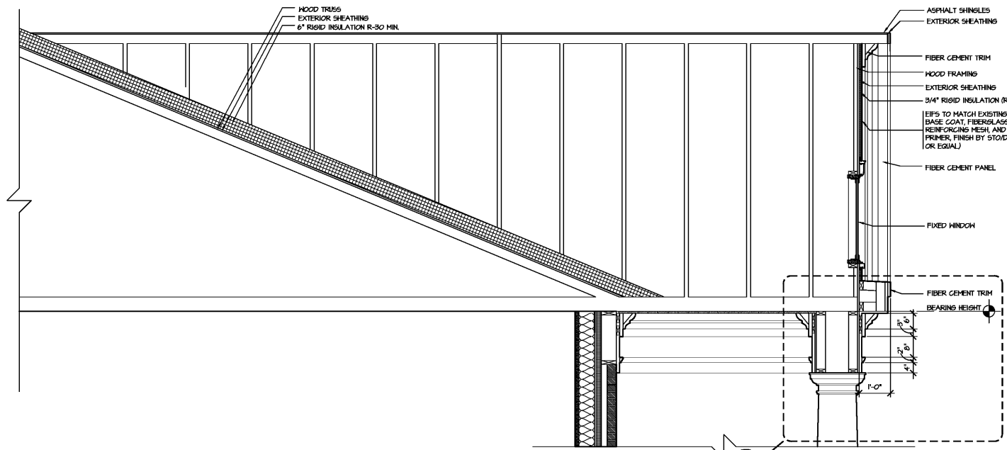
1 WALL SECTION SCALE: 1/2" = 1'-0"
