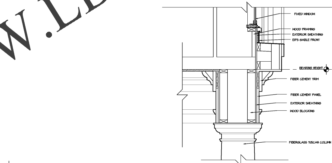
5 PORCH COLUMN DETAIL SCALE: 1" = 1'-0"
