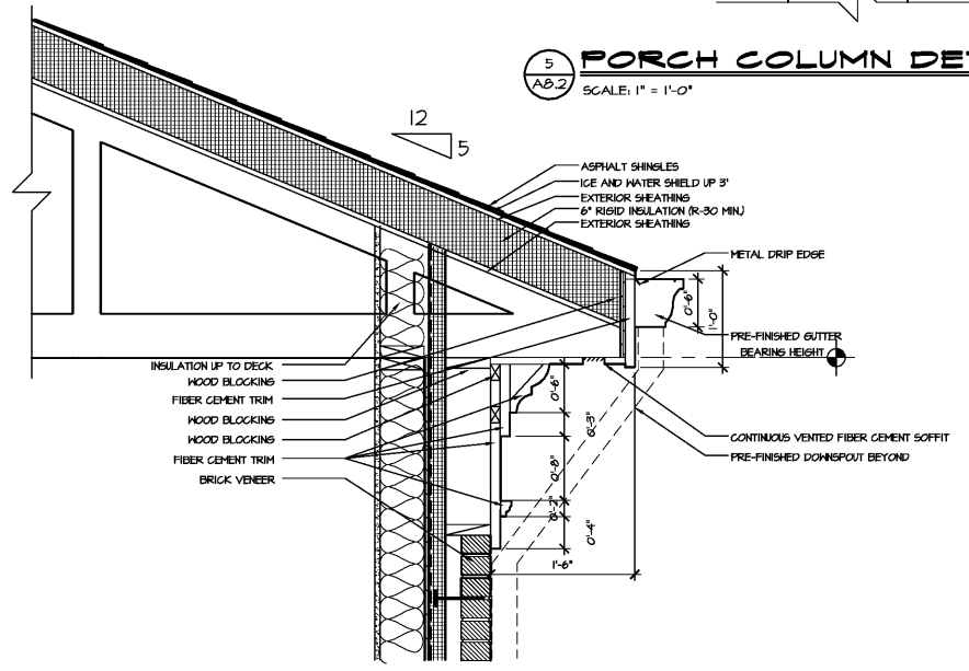
6 EAVE DETAIL SCALE: 1" = 1'-0"
