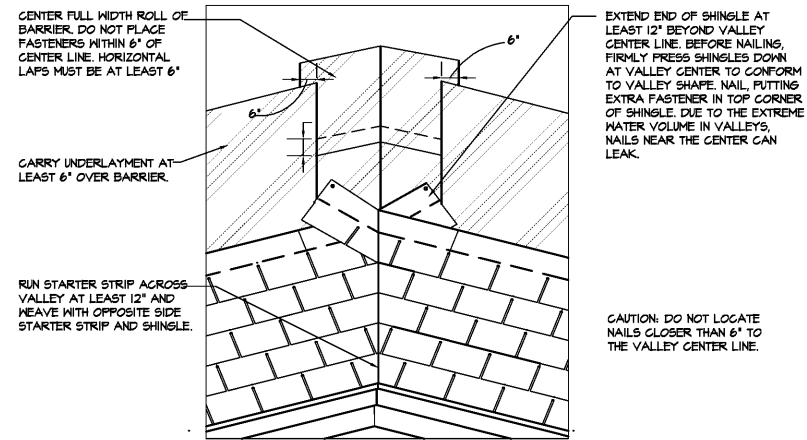
1 SHINGLE VALLEY DETAIL A4.3 SCALE: N.T.S.
