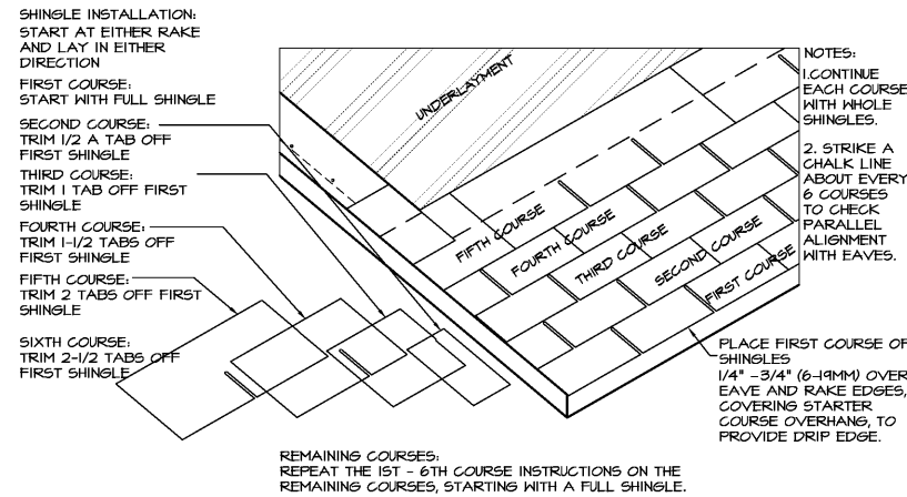
2 SHINGLE TYP. INSTALLATION A4.3 SCALE: N.T.S.
