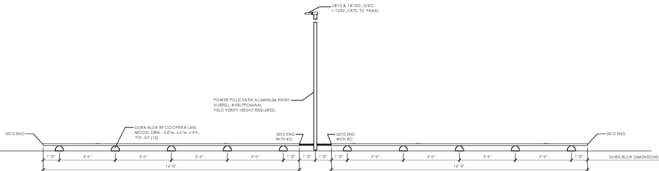
D3 Gondola Lighting Raceway Detail SCALE: N.T.S.
