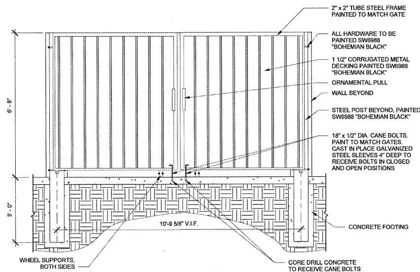
6 DUMPSTER GATE ELEVATION A-402 SCALE: 1/2" = 1'-0"
