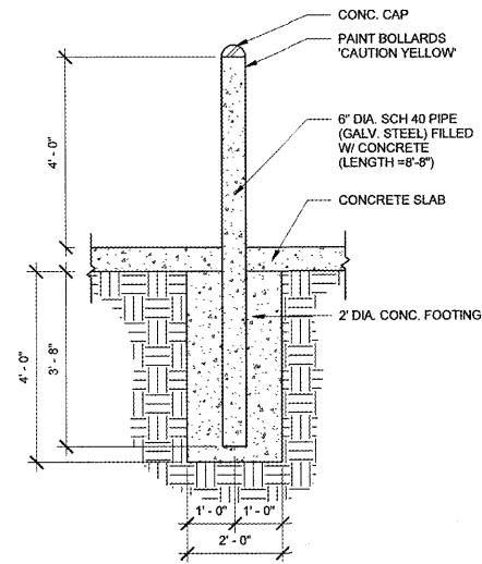
7 DUMPSTER BOLLARD DETAIL A-402 SCALE: 1/2" = 1'-0"
