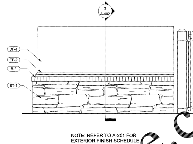
2 DUMPSTER ENCLOSURE ELEVATION A-402 SCALE: 1" = 1'-0"
