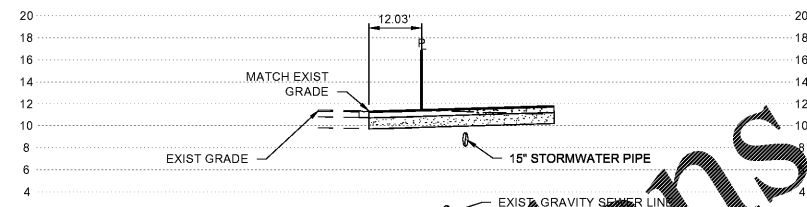
SECTION D-D
