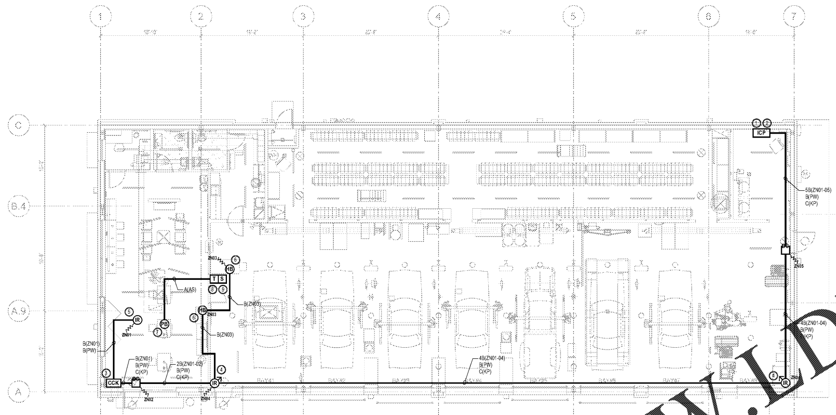
INTRUSION ALARM PLAN SCALE: 1/8" = 1'-0"
