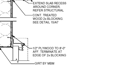
14 O.H. DOOR THRESHOLD A6 SCALE: 1"=1'-0"
