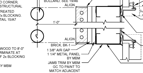
15 SECTION @ T.O. WALL A6 SCALE: 1 1/2"=1'-0"
