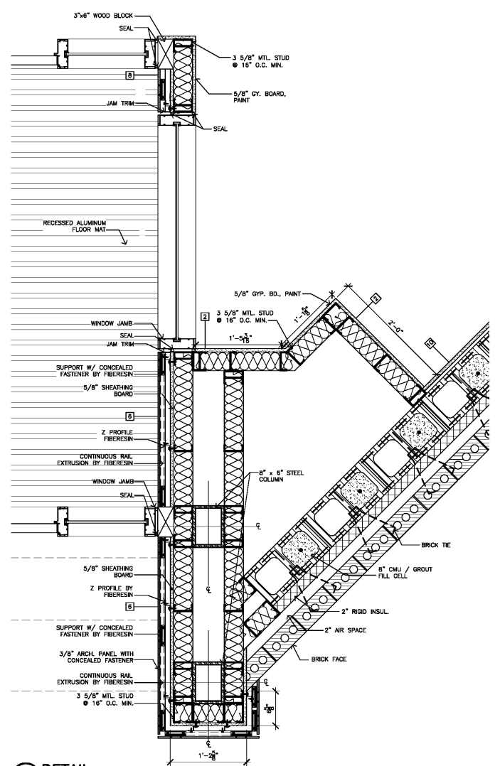
1 DETAIL SCALE: 1"=1'-0"
