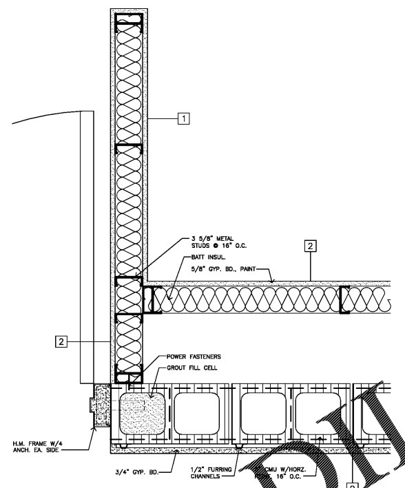
4 DETAIL SCALE: 1 1/2"=1'-0"
