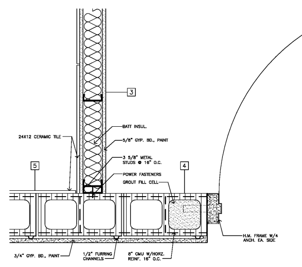
3 DETAIL SCALE: 1 1/2"=1'-0"
