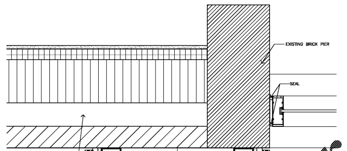
1 DETAIL SCALE: 1"=1'-0"
