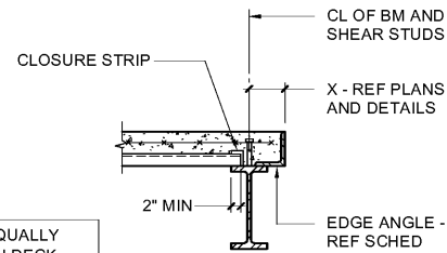
EDGE PERPENDICULAR
