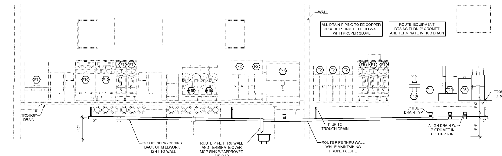
2 EQUIPMENT DRAIN ELEVATION SCALE: N.T.S.
