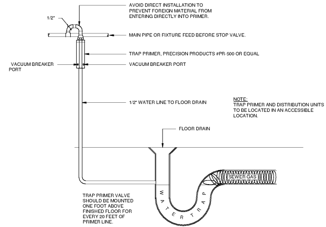
TRAP PRIMER NO SCALE
