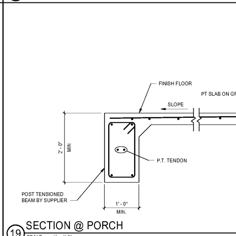
19 SECTION @ PORCH SCALE: 1" = 1'-0"
