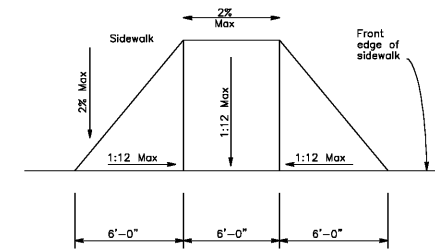
CONCRETE FLARED RAMP DETAIL N.T.S.
