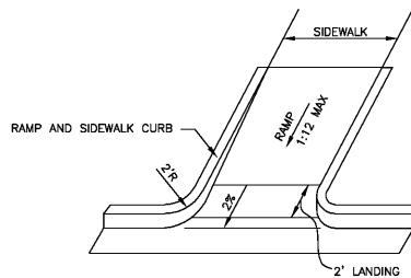
CURB RETURN RAMP DETAIL N.T.S.
