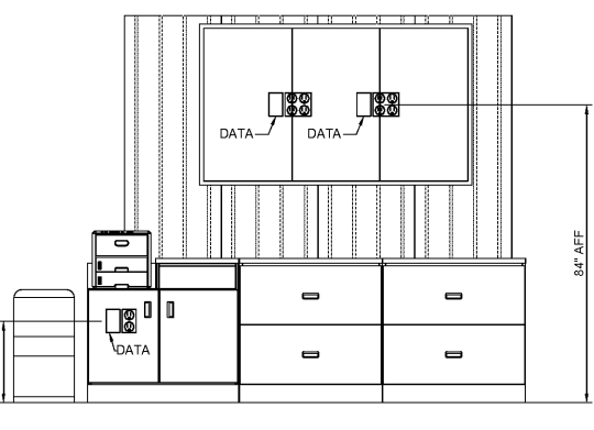
9 E4 DISPLAY SCREENS DETAIL SCALE: NONE
