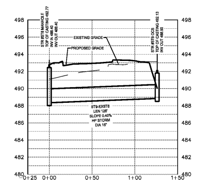
ST9-ST8 Horizontal Scale: 1" = 40' Vertical Scale: 1" = 4'
