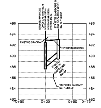
ST2B-ST2 Horizontal Scale: 1" = 40' Vertical Scale: 1" = 4'
