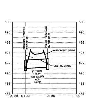
ST17-ST16 Horizontal Scale: 1" = 40' Vertical Scale: 1" = 4'
