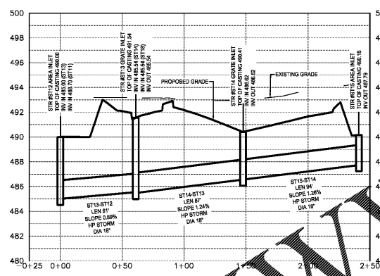
ST15-ST12 Horizontal Scale: 1" = 40' Vertical Scale: 1" = 4'
