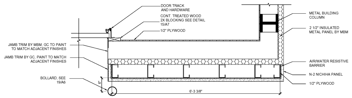
4 PLAN DETAIL A1.2 SCALE: 1"=1'-0"
