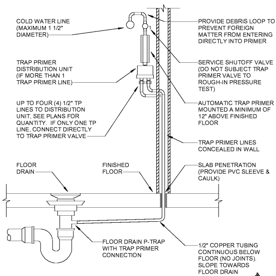
4 AUTOMATIC TRAP PRIMER P0.3 N.T.S.
