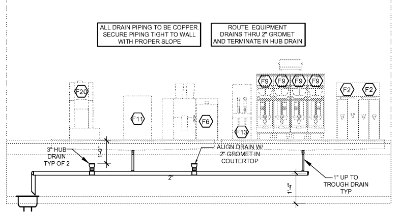
2 EQUIPMENT DRAIN ELEVATION SCALE: N.T.S.
