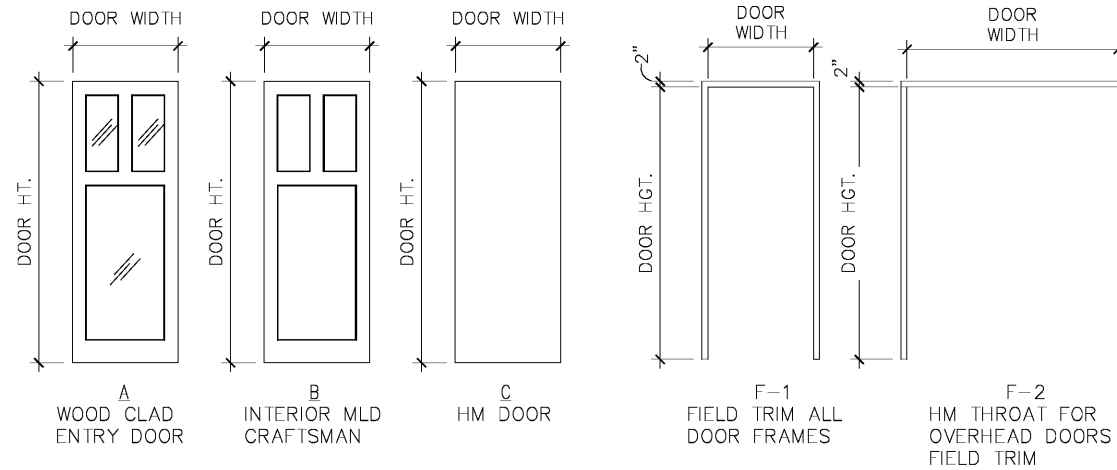
DOOR TYPES
