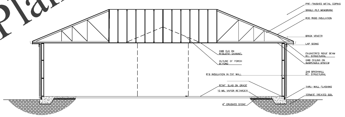
1 SECTION SCALE: 1/4"=1'-0"
