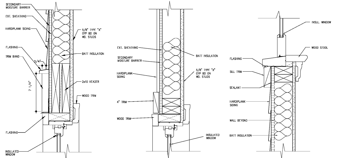
3 DETAIL: Window Head SCALE: 3"=1'-0" 2 DETAIL: Window Jamb SCALE: 3"=1'-0" 1 DETAIL: Window Sill SCALE: 3"=1'-0"
