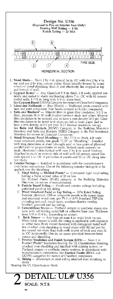
2 DETAIL: UL# U356 SCALE: N.T.S.
