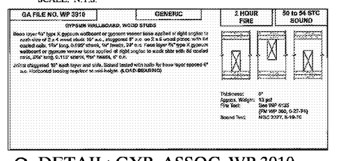
8 DETAIL: GYP. ASSOC. WP 3910 SCALE: N.T.S.
