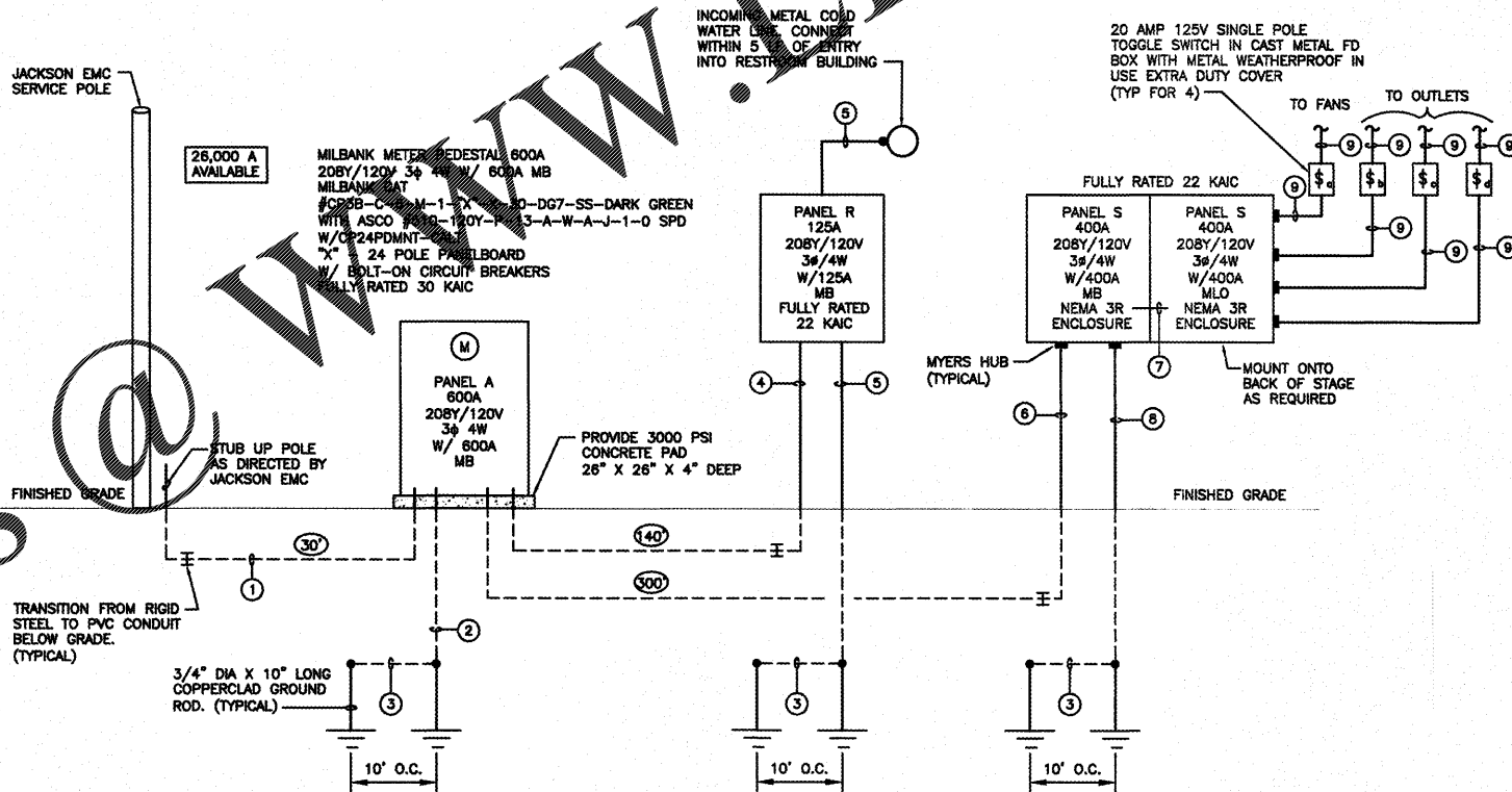
2 POWER RISER DIAGRAM E-5 SCALE: NTS
