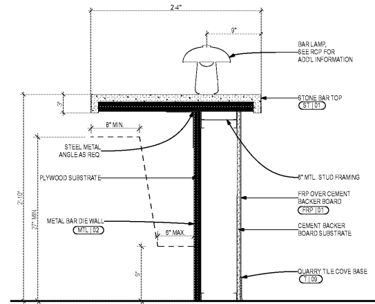
4 BAR ADA SECTION SCALE: 1 1/2\"/>
