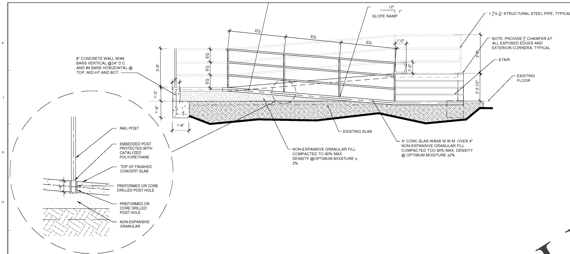
F1 INTERIOR CONCRETE RAMP SECTION 1/2"=1'-0"
