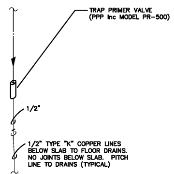
TRAP PRIMER PIPING DIAGRAM NO SCALE
