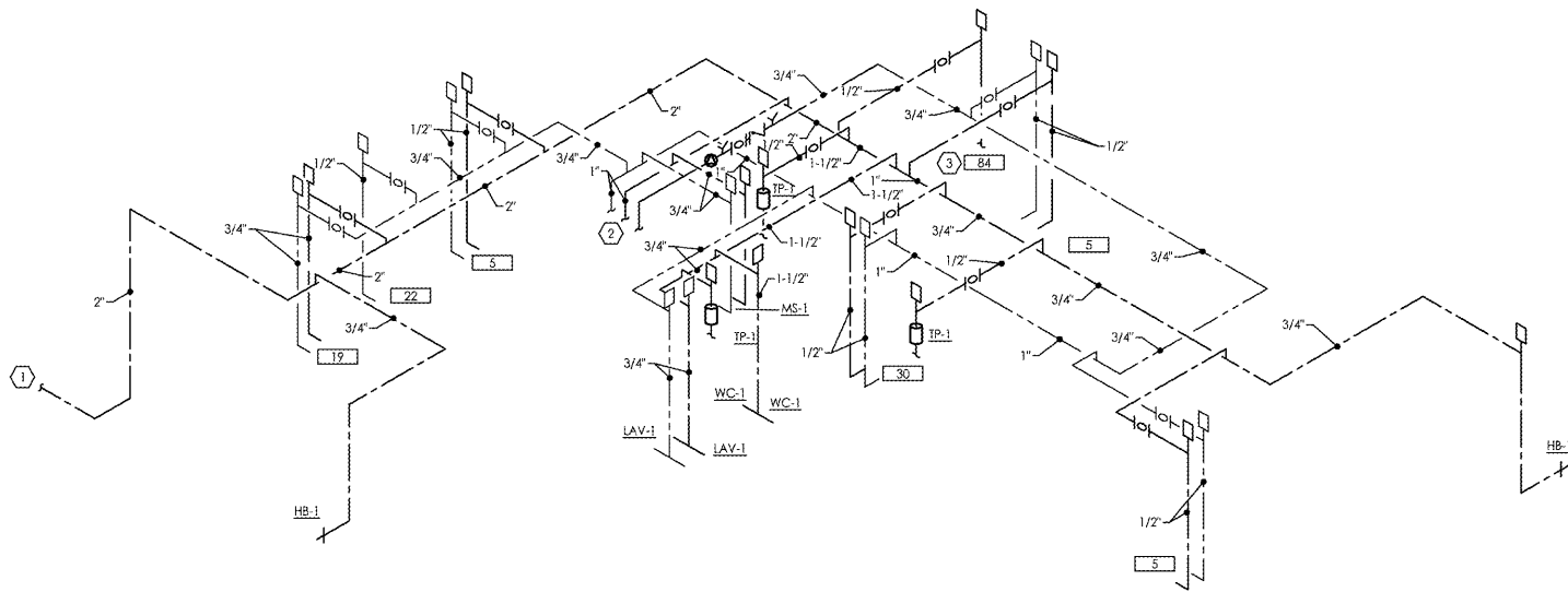
3 WATER RISER DIAGRAM N.T.S.
