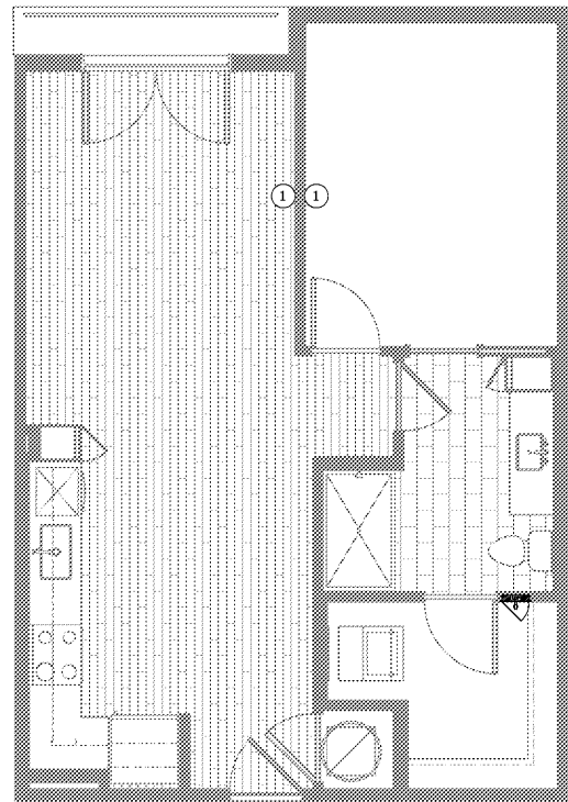
1 UNIT A3.1 1/4" = 1'-0"
