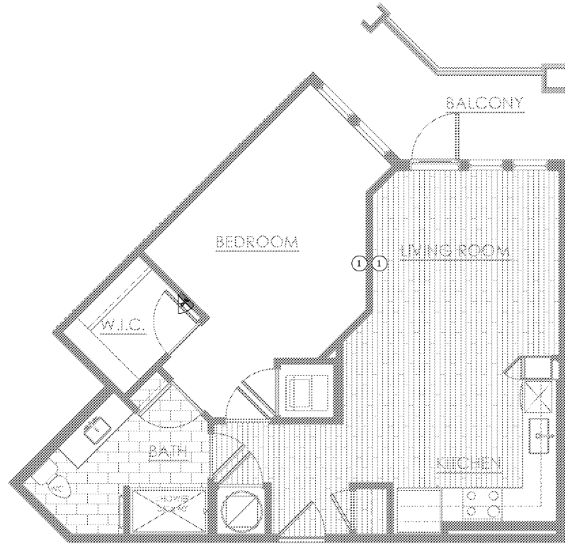
2 UNIT A4 1/4" = 1'-0"
