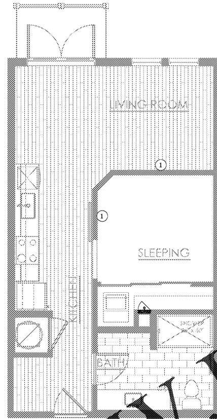
3 UNIT A1 14'4" x 12'
