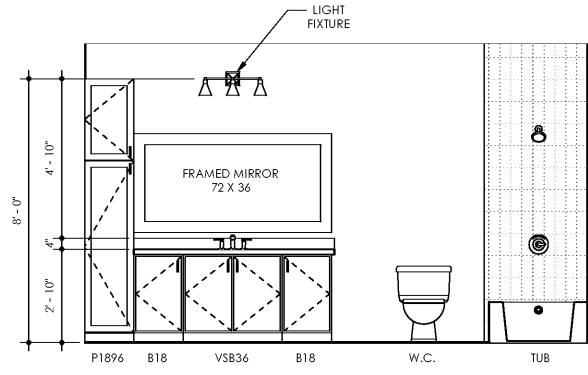
15 BATH UNIT C1-A SCALE: 3/8" = 1'-0"
