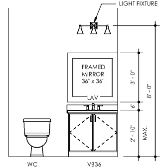
1 BATH UNITS C3 SCALE: 3/8" = 1'-0"
