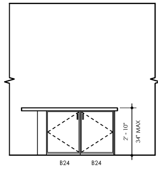
7 KITCHEN UNIT B5-A SCALE: 3/8" = 1'-0"
