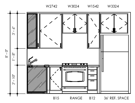
4 KITCHEN UNIT A4-A SCALE: 3/8" = 1'-0"
