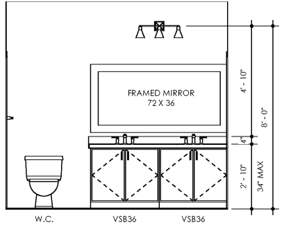
14 BATH UNIT C1-A SCALE: 3/8" = 1'-0"
