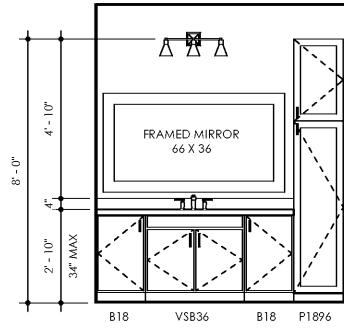
10 BATH UNIT B5-A SCALE: 3/8" = 1'-0"
