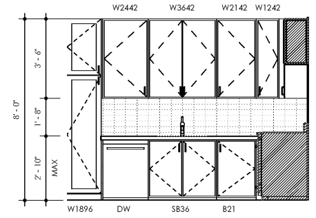
5 KITCHEN UNIT A4-A SCALE: 3/8" = 1'-0"
