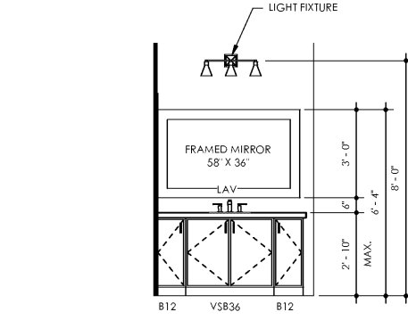
4 BATH UNIT S2 SCALE: 3/8" = 1'-0"
