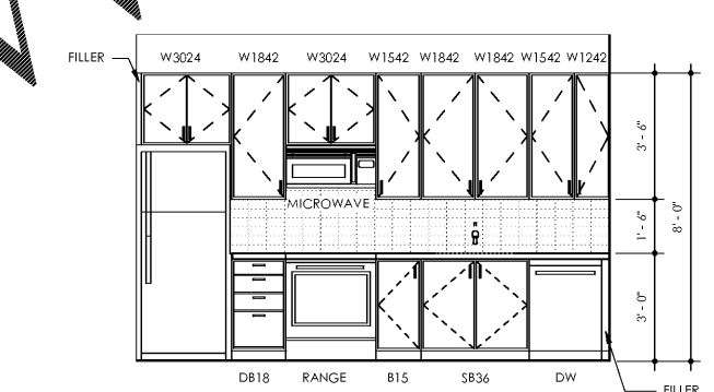
5 KITCHEN UNITS A1 SCALE: 3/8" = 1'-0"
