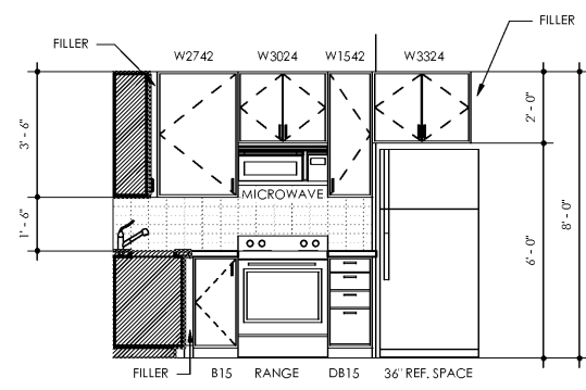
13 KITCHEN UNITS A4 SCALE: 3/8" = 1'-0"
