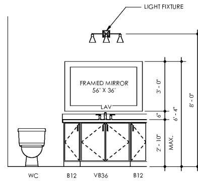
14 BATH UNITS A4 SCALE: 3/8" = 1'-0"
