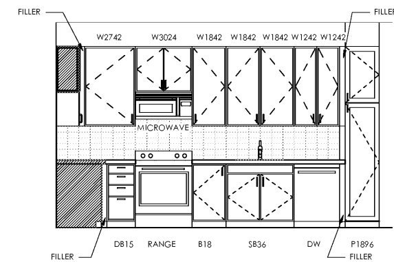
10 KITCHEN UNITS A3, A3.1 SCALE: 3/8" = 1'-0"
