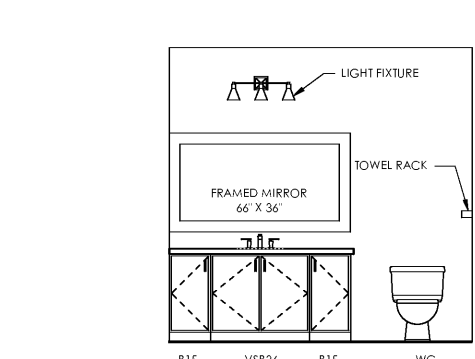
8 BATH UNIT A2 SCALE: 3/8" = 1'-0"
