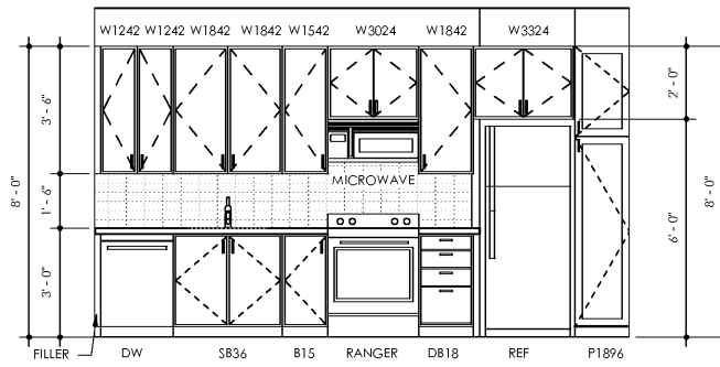
7 KITCHEN UNITS A2 SCALE: 3/8" = 1'-0"
