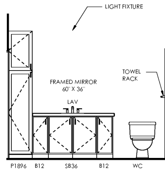
11 BATH UNITS A3, A3.1 SCALE: 3/8" = 1'-0"
