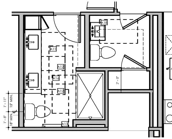
8 BATH UNIT B5 SCALE: 3/8" = 1'-0"
