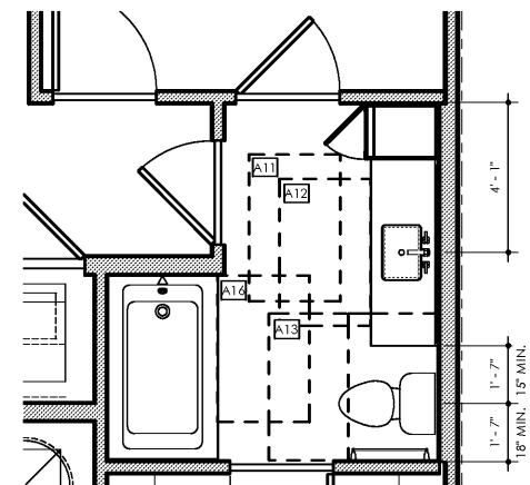
3 BATH UNITS B3, B4 SCALE: 3/8" = 1'-0"
