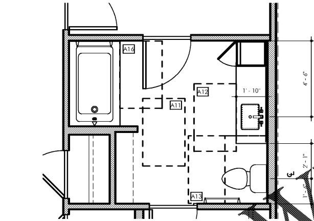
7 BATH UNIT B5 SCALE: 3/8" = 1'-0"
