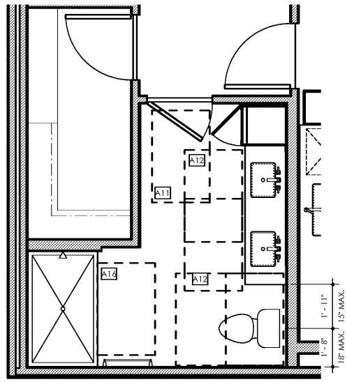
10 BATH UNIT B6 SCALE: 3/8" = 1'-0"
