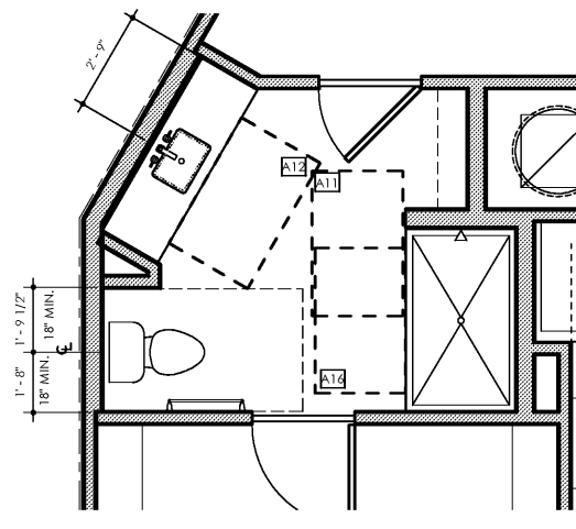
5 BATH UNIT B4 SCALE: 3/8" = 1'-0"
