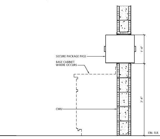
4 PACKAGE BOX SECTION SCALE: 1" = 1'-0"
