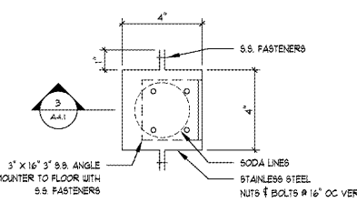
8 A4.1 SODA LINE WRAP DETAIL SCALE: 3"=1'-0"
