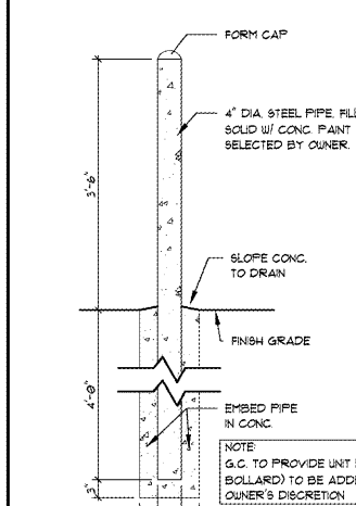
9 A4.1 BOLLARD SECTION SCALE: 3"=1'-0"
