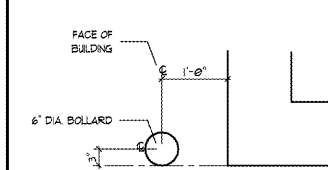
10 A4.1 BOLLARD DETAIL SCALE: 3"=1'-0"
