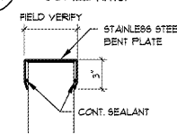
2 A4.1 DRIVE THRU LOOP DIAGRAM DETAIL SCALE: N.T.S.
