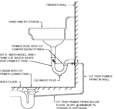
3 TRAP PRIMER DETAIL
