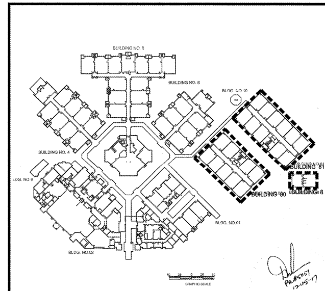
1 KEY PLAN SCALE: 1" = 100'-0"
