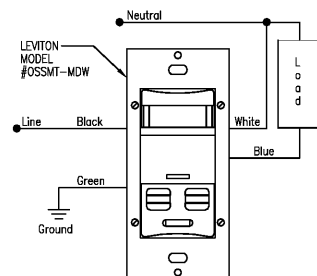
3 "A" OCCUPANCY SENSOR N.T.S.
