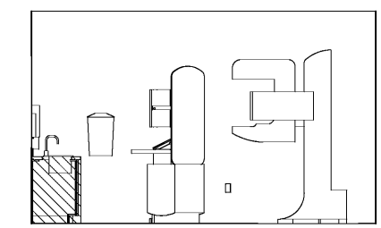
2 MAMMO - E 3/8" = 1'-0"
