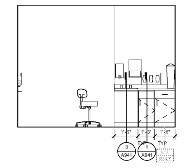
1 MAMMO - N 3/8" = 1'-0"
