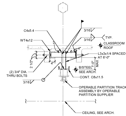
3 SECTION SCALE: 3/4" = 1'-0"
