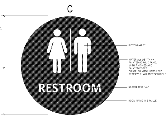
7 RESTROOM ID 3 Scale: Half
