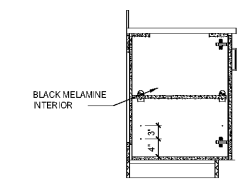
13K SECTION SCALE: 1/4" = 1'-0"
