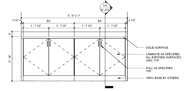
13E ELEVATION SCALE: 3/4" = 1'-0"
