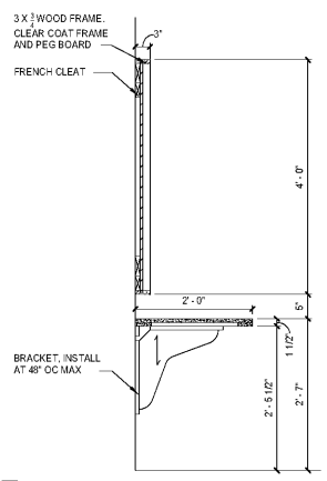
7K SECTION SCALE: 3/4" = 1'-0"
