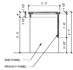
1K SECTION SCALE: 3/4" = 1'-0"
