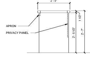
4K ELEVATION SCALE: 3/4" = 1'-0"
