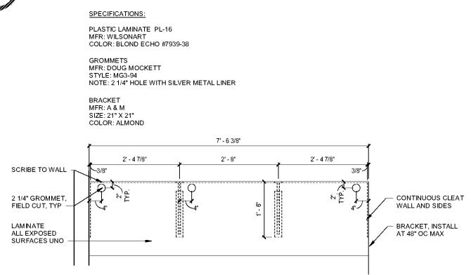
7E ELEVATION SCALE: 3/4" = 1'-0"
