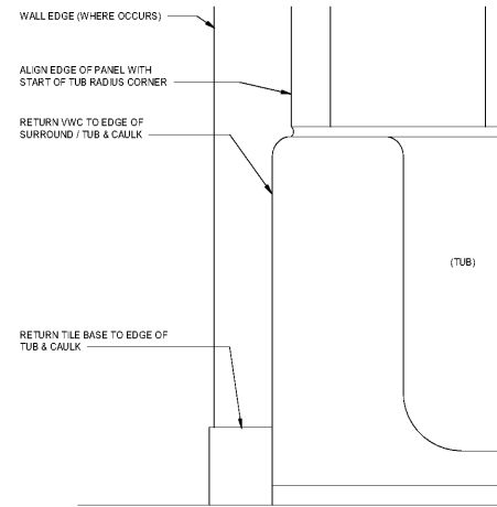
8 TUB SURROUND EDGE SCALE: 3" = 1'-0"
