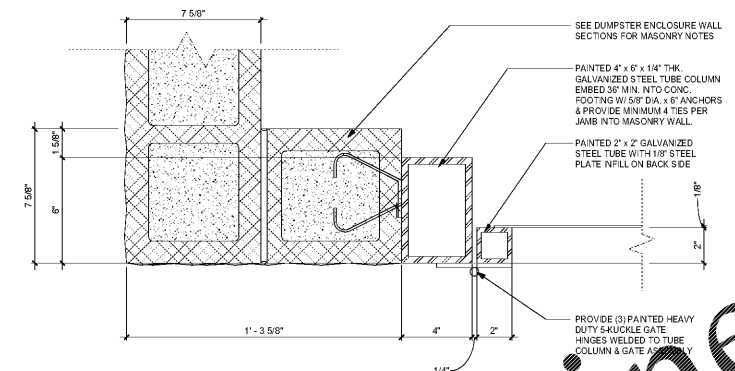
A JAMB DETAIL SCALE: 3" = 1'-0"
